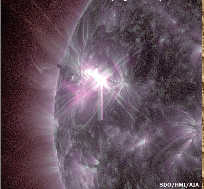
M2.4 Solar Flare (Region 2277)
