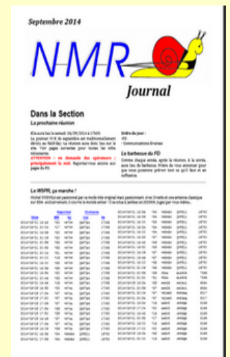
NMR 09/2014
